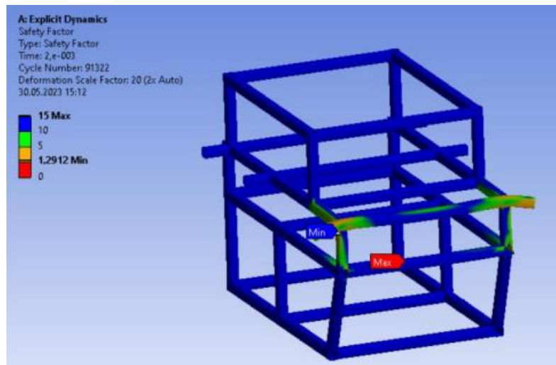
Şekil 9. Çarpışma Analizi Sonucu Şaside Oluşan Güvenlik Kat Sayısı
