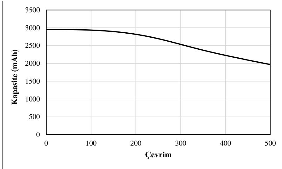
Şekil 5. Deşarj kapasitesinin çevrime bağlı değişim grafiği
