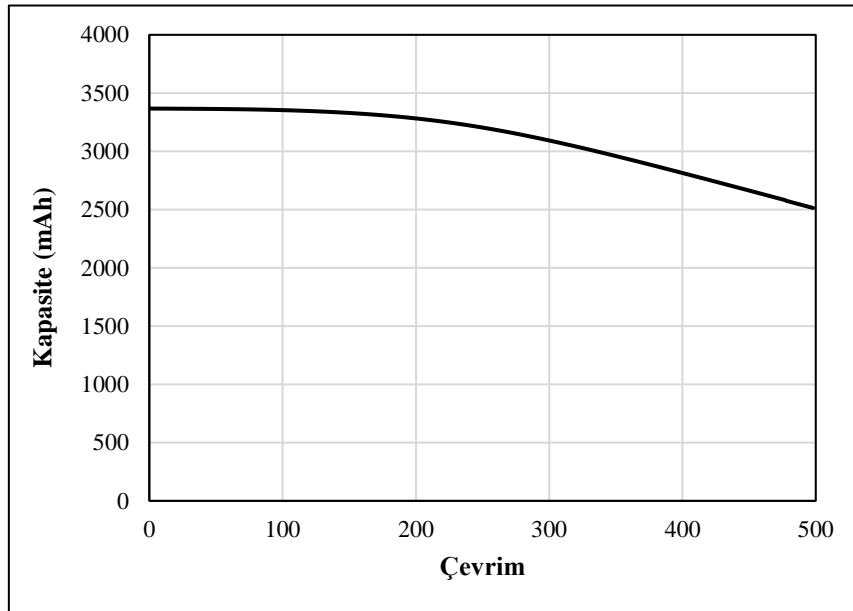
Şekil 4. Şarj kapasitesinin çevrime bağlı değişim grafiği
