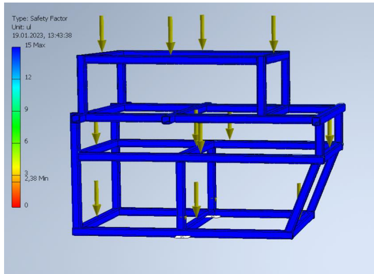
Şekil 5. Şasi Güvenlik Faktörü
