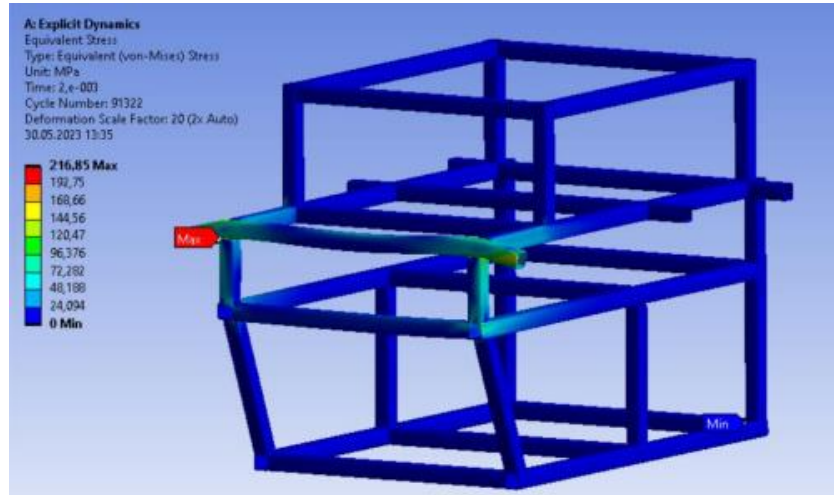
Şekil 8. Maksimum Von Mises Gerilmeleri
