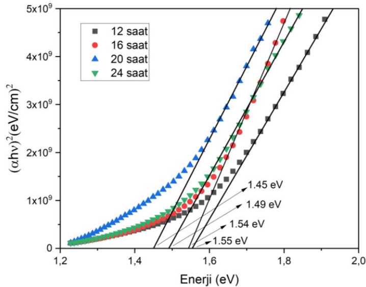
Şekil 2.4. Farklı sentez sürelerinde elde edilmiş CuO ince filmlerin (\alpha h\nu)^2 -Enerji grafikleri
