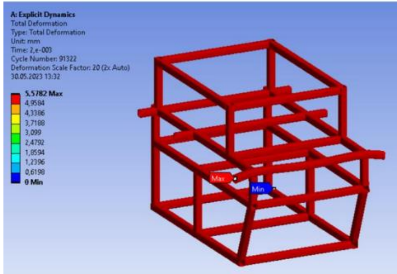
Şekil 7. Çarpışma Analizi Sonucu Oluşan Toplam Yer Değiştirme Sonuçları
