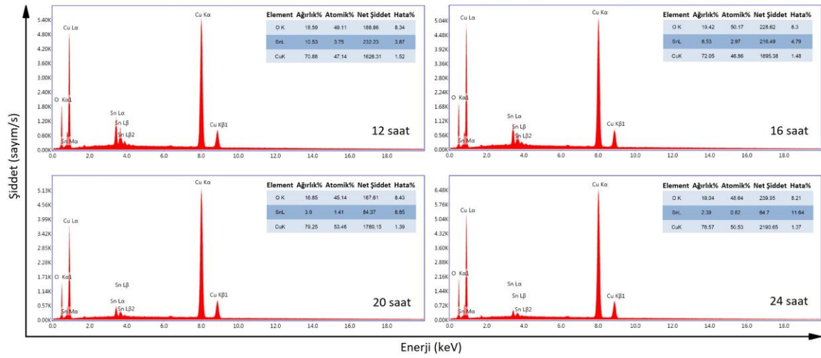
Şekil 2.3. Farklı sentez sürelerinde büyütülen CuO ince filmlerin EDAX spektrumları
