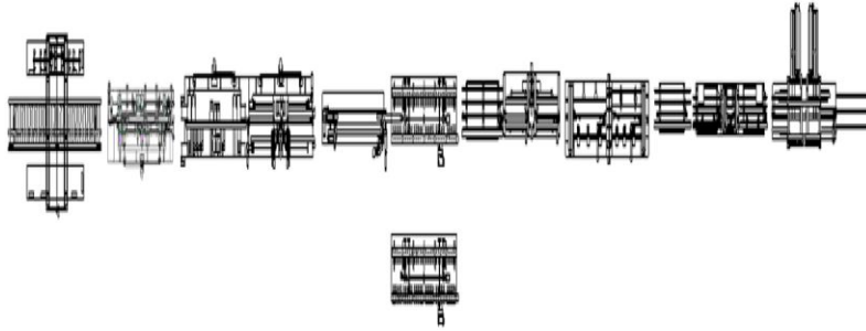
Şekil 1. 3. Üretim hattı layout
