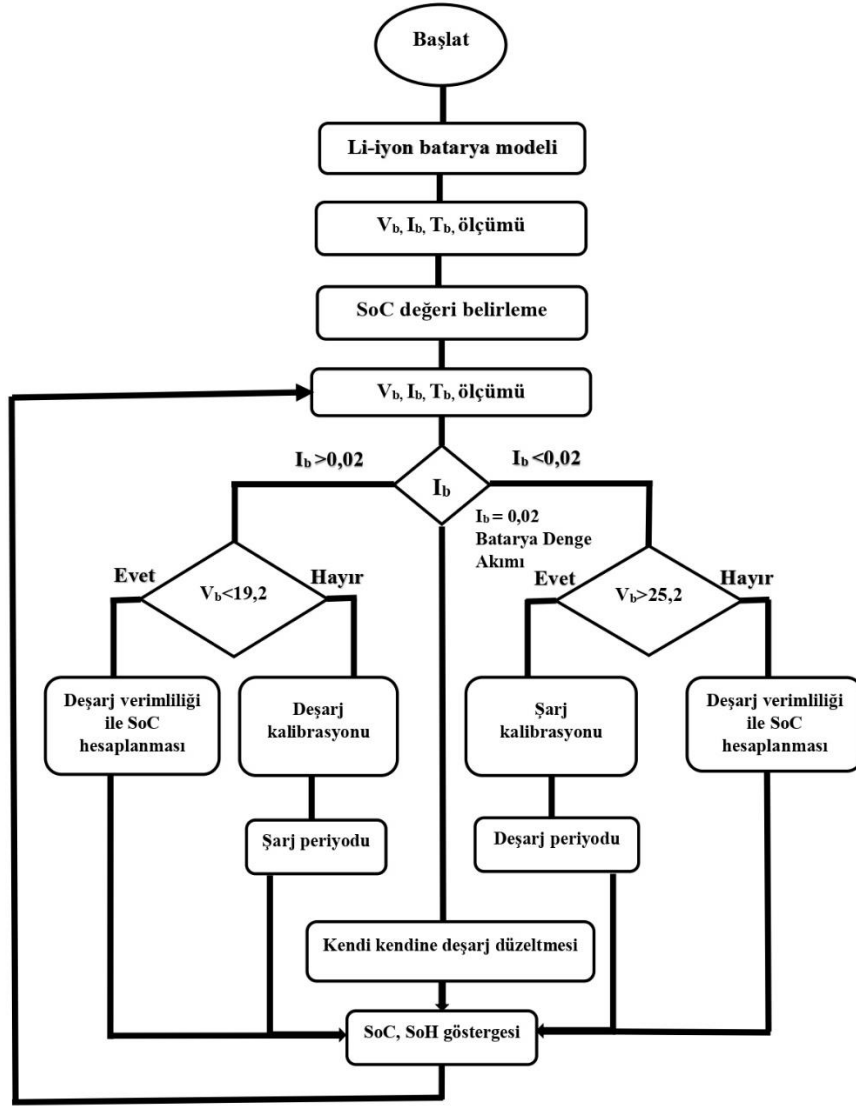
Şekil 3. Şarj döngü ömrü belirleme algoritması
