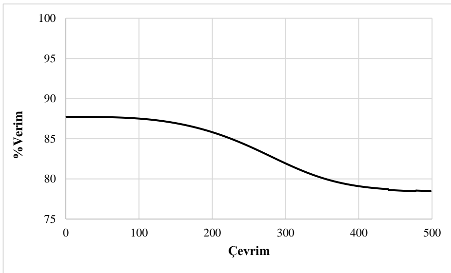
Őekil 6. evrim sayısına baęlı batarya verimi
