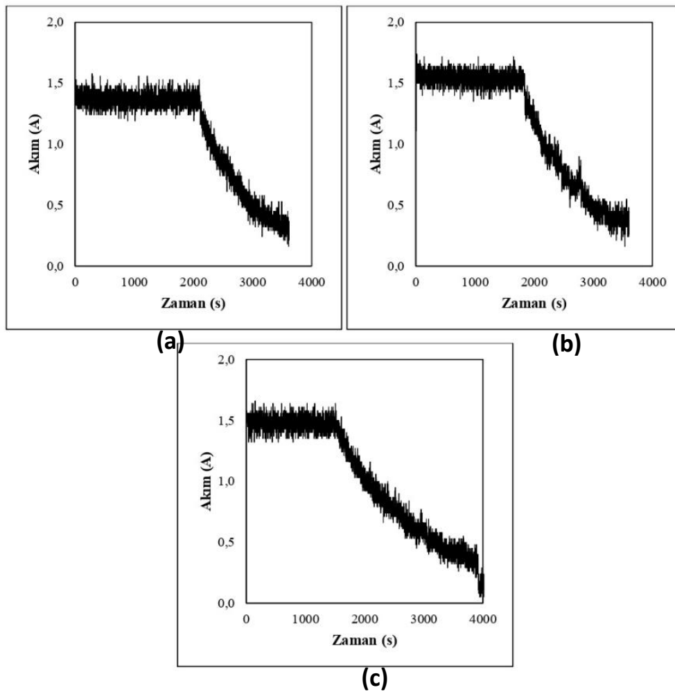
Şekil 7. Çevrimlere baęlı şarj profili grafikleri; a: 1. Çevrim, b: 250. Çevrim, c: 500. Çevrim
