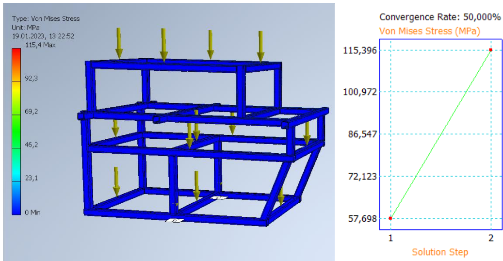
Şekil 3. Şasi Von Mises Gerilmesi
