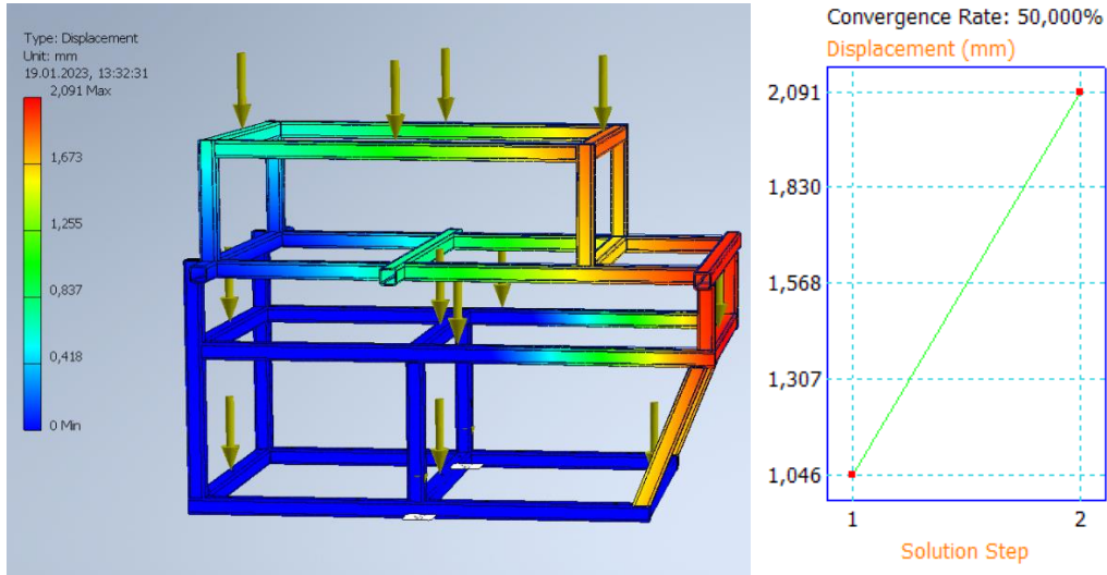
Şekil 4. Şasi Yer değıştirme Miktarı
