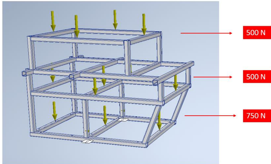
Şekil 2. TİKA gövde tasarımı ve uygulanan kuvvetler.
