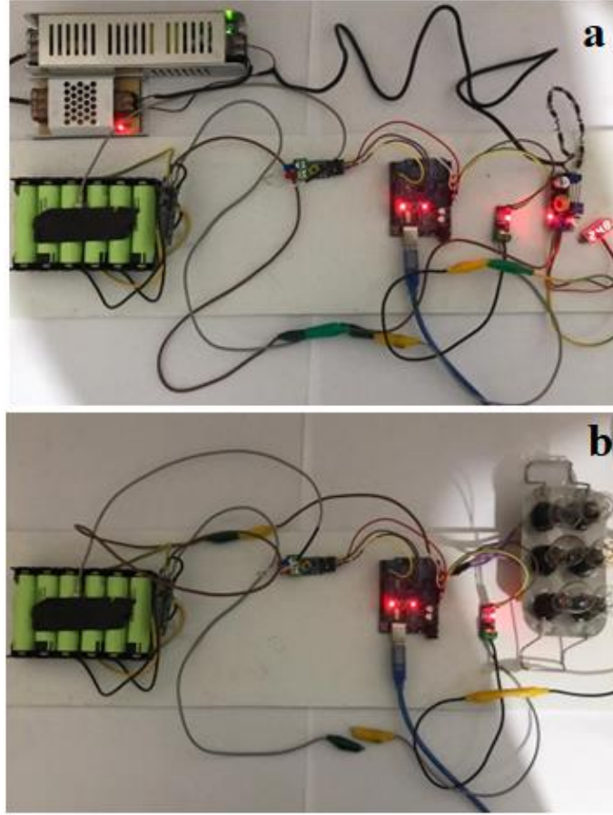
Şekil 1. (a) Şarj, (b)deşarj akım sayma devresi
