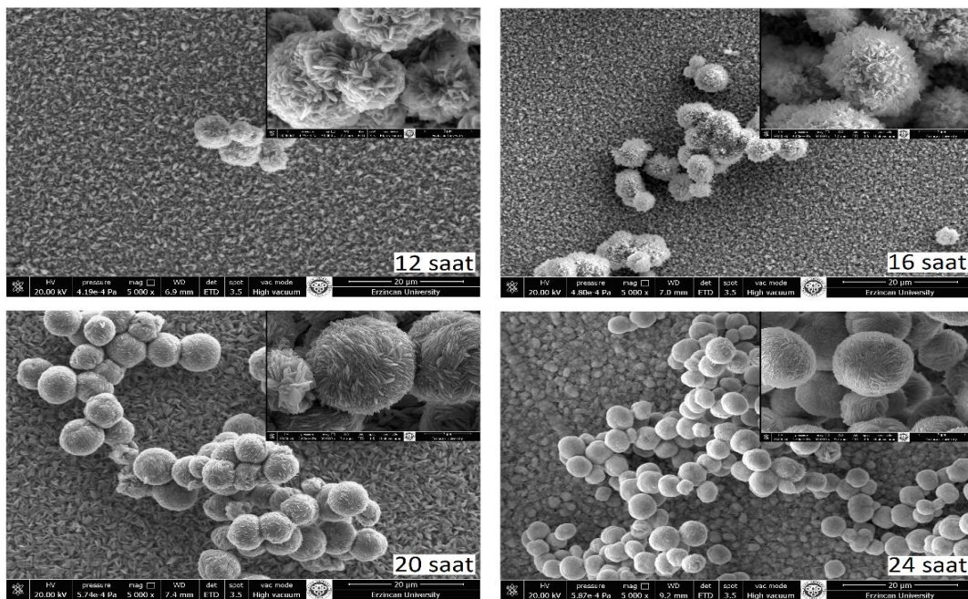
Şekil 2.2. Farklı reaksiyon sürelerinde büyütülen CuO ince filmlerin SEM görüntüleri
