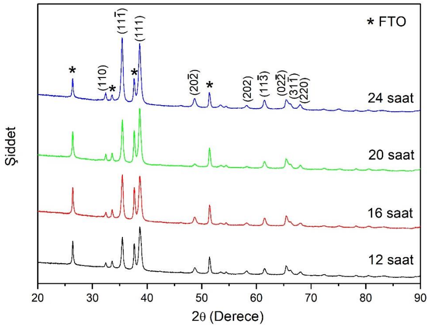
Şekil 2.1. Farklı reaksiyon sürelerinde büyütülen CuO ince filmlerin XRD desenleri
