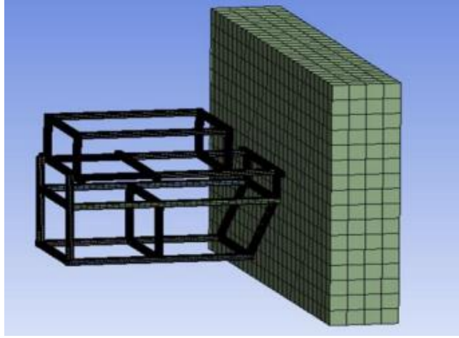
Şekil 6. Çarpışma Analizi Mesh Görünümü
